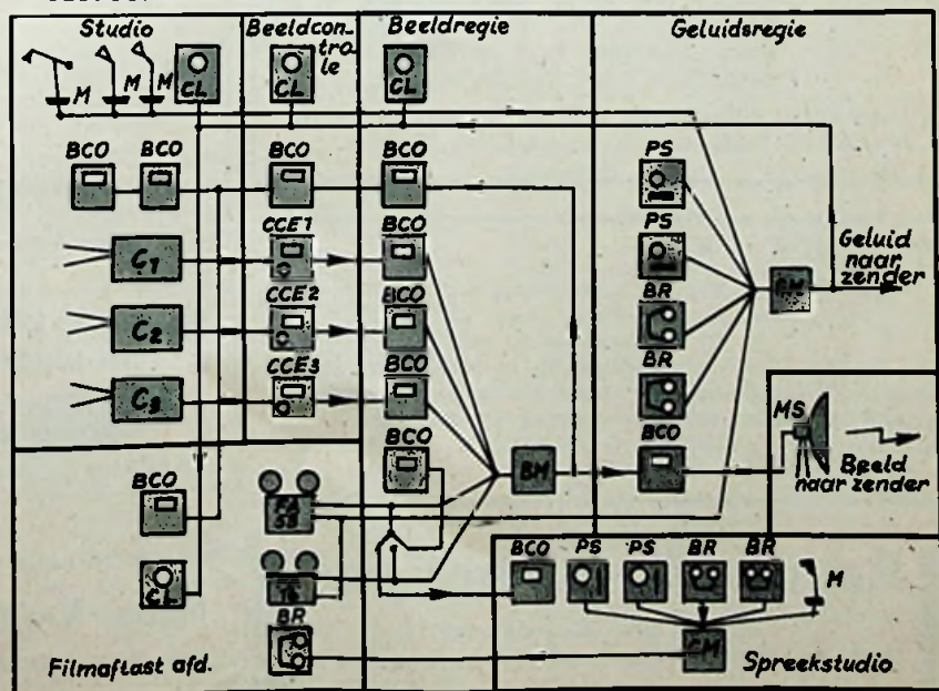
BLOKSCHEMA VAN DE ELECTR. INRICHTING IN DE TELEVISIESTUDIO
