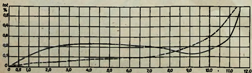
Distorsiecurve voor AM-buizen (volle lijn) en Europese type, in beide gevallen is d_{100} minder dan 0,3 procent.
